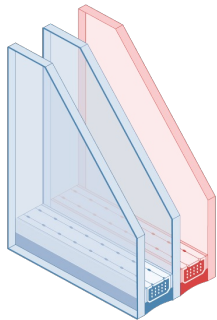
Hergebruikt origineel pakket + derde laag nieuw gecoat
