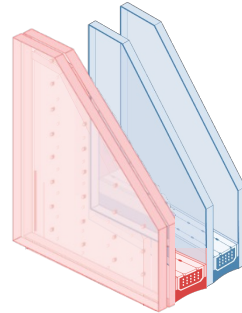
Hergebruikt origineel pakket + derde laag vacuümglas
