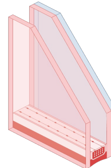
Dakraam met 50% circulair gelamineerd binnenblad
