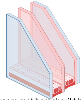
Dakraam met hergebruikt buitenblad + 50% circulair gelamineerd binnenblad
